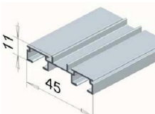
FP-6600 kattoon/seinään; kaksiurainen kisko
