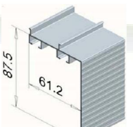
FP-6607 kattoon/seinään; kaksiurainen otsalaudalla
