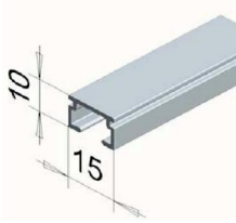
FP 6100 kattoon/seinään; yksiurainen verhokisko
