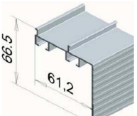
FP-6606 kattoon/seinään, kaksiurainen otsalaudalla
