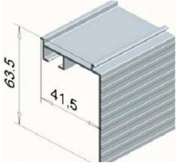
FP-6106 kattoon/seinään; Yksiurainen verhokisko laudalla
