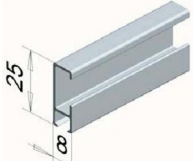
FP-6400 kattoon/seinään; yksiurainen verhokisko
