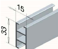
FP-6200 Kattoon/seinään; järeä väliverhokisko
